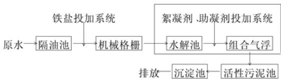
附图 工艺流程图
