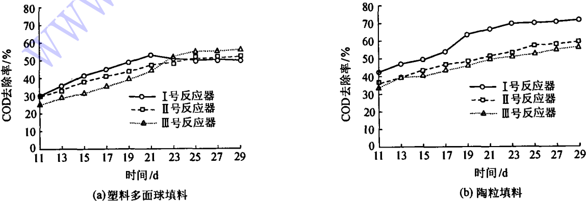
图2 挂膜效果曲线
