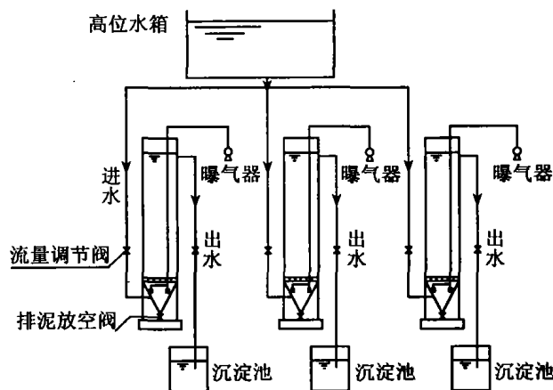
图 1 试验装置流程
