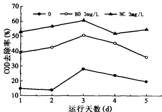
图6 低气水比条件下COD的去除效果
