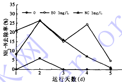
图9 未曝气条件下NH 3 -N的去除效果
