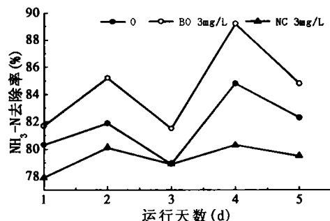
图5 最佳气水比条件下 \text{NH}_3\text{-N} 的去除效果
