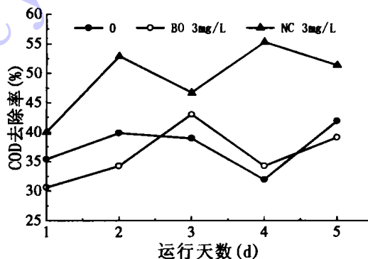
图4 最佳气水比条件下 COD 的去除效果
