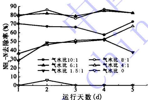
图3 不同气水比条件下 \text{NH}_3\text{-N} 的去除效果
