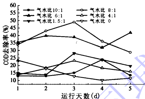
图2 不同气水比条件下 COD 的去除效果
