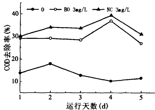
图8 未曝气条件下COD的去除效果
